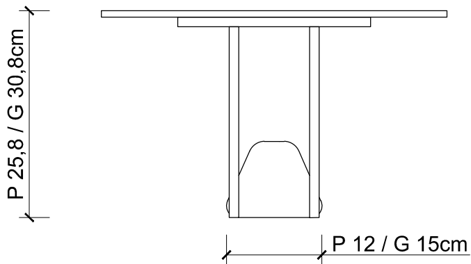
Vista Lateral
