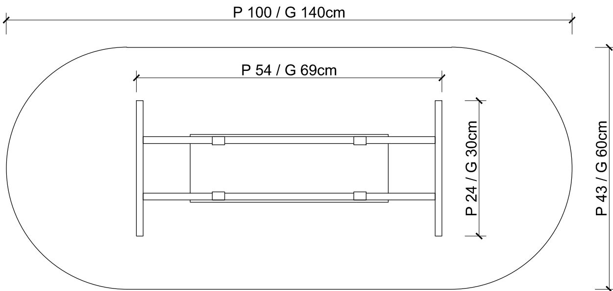
Vista superior
