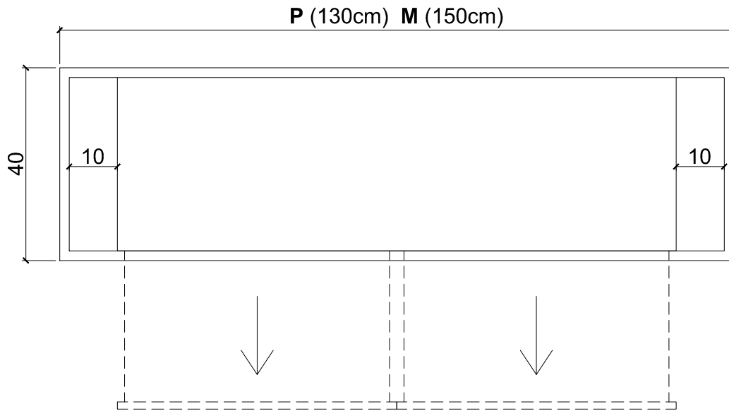
Vista superior
