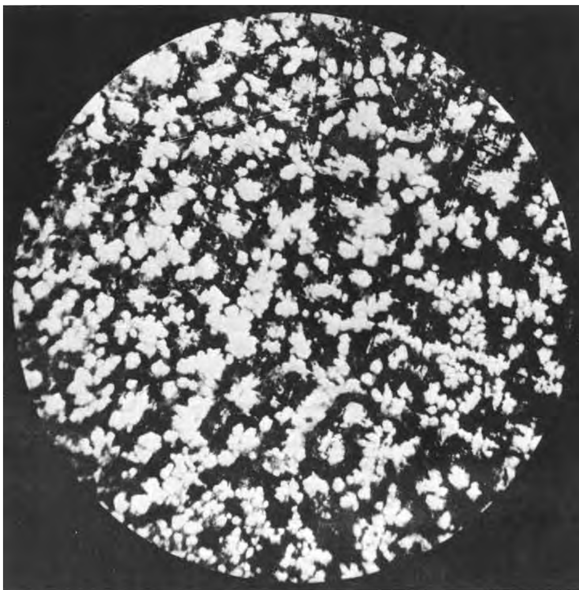
FIGURA 9.1 Microfotografia de uma secção da fateixa de cobre pertencente ao barco de Quéops em Gizeh.
