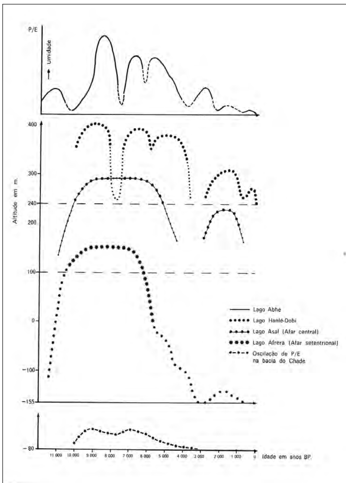
FIGURA 16.7 Variações dos níveis lacustres nas bacias do Afar. As curvas relativas aos lagos Abhé, Hanlé-Dobi e Asal, situados no Afar central, estão representadas no mesmo gráfico. A do lago Afrera é independente. Pode-se estabelecer comparação com a curva de oscilação de P/E na bacia do Chade (segundo F. Gasse, 1975).
