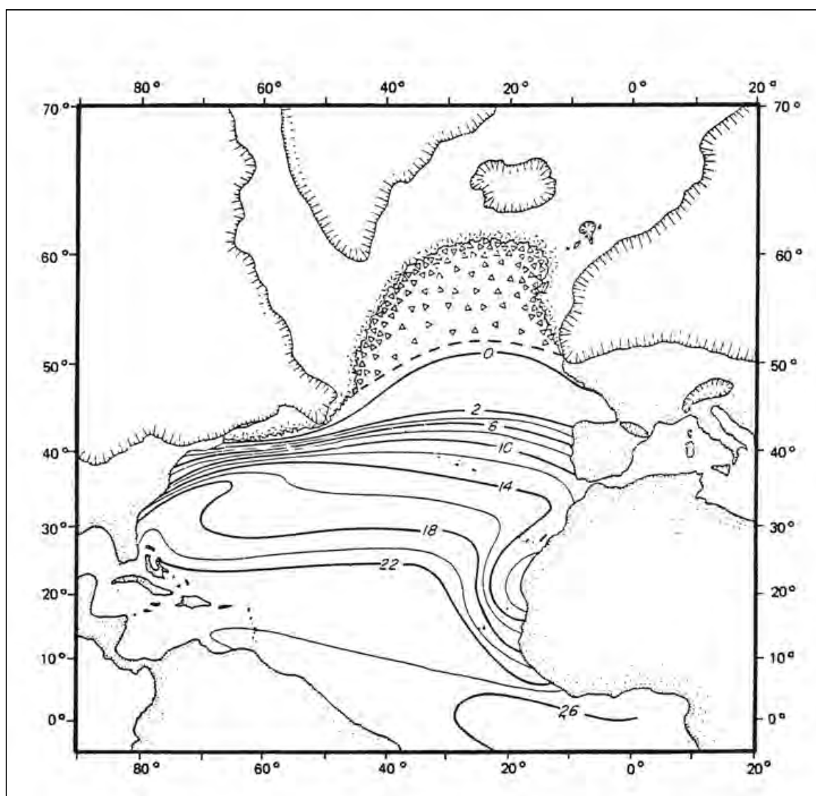
FIGURA 16.3 Mapa das isotermas da água de superfície do oceano Atlântico em fevereiro, 18000 B.P. As isotermas em pontilhado são interpretativas. As grandes massas de gelo continental são delineadas por contornos hachurados; a banquisa permanente por contornos granulados. A linha de costa glacial é traçada para um nível do mar inferior em 85 m ao atual (segundo Mc Intyre et alii , 1975).
