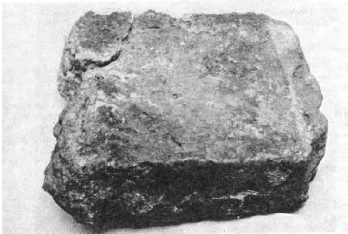
FIGURA 9.3 Bloco de vitrificação mostrando a superfície superior plana, as paredes laterais e uma parte do cadinho ainda aderente ao lado direito.
