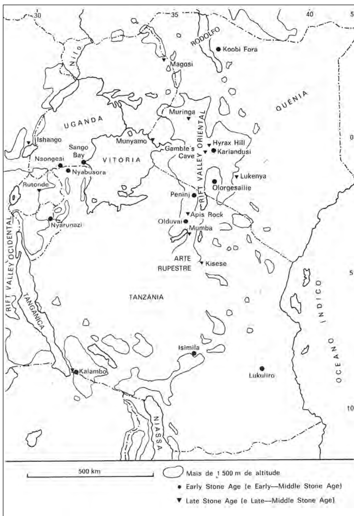
FIGURA 19.2 África oriental: principais jazidas da Idade da Pedra (1974).
