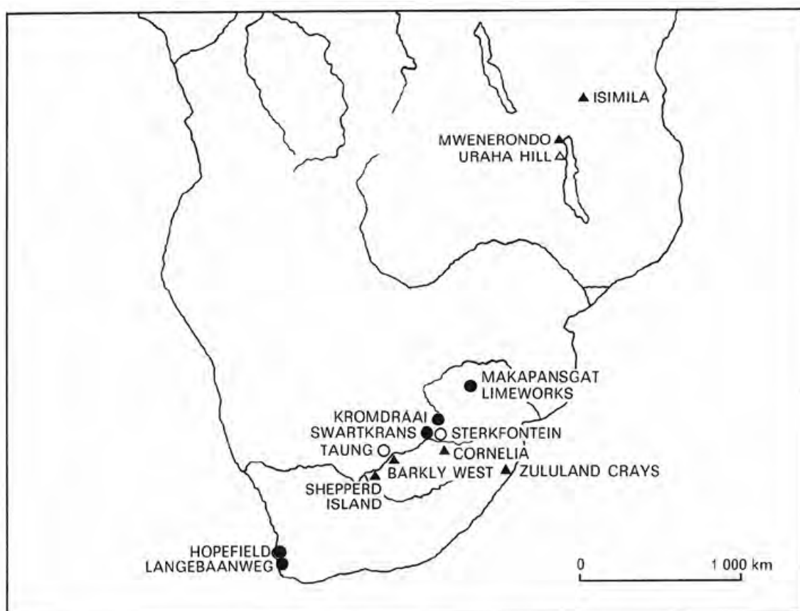
FIGURA 20.3 Principais depósitos de fauna e fósseis humanos do fim do Plioceno (fauna = \triangle ; fósseis humanos = \circ ) ao início do Pleistoceno ( \blacktriangle ; \bullet ) na África austral ( Apud CLARK, J. D. The Prehistory of Africa . Londres, Thames and Hudson, 1970. Figs. 9).
