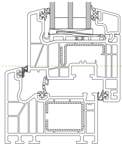
Herkömmliche Balkon-/Terrassentür mit umlaufendem Blendrahmen
