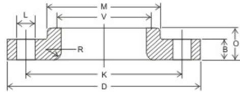
Flange solto
