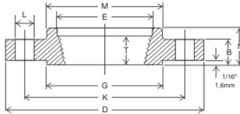
Flange roscado
