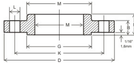
Flange sobreposto
