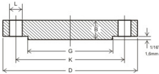
Flange cego
