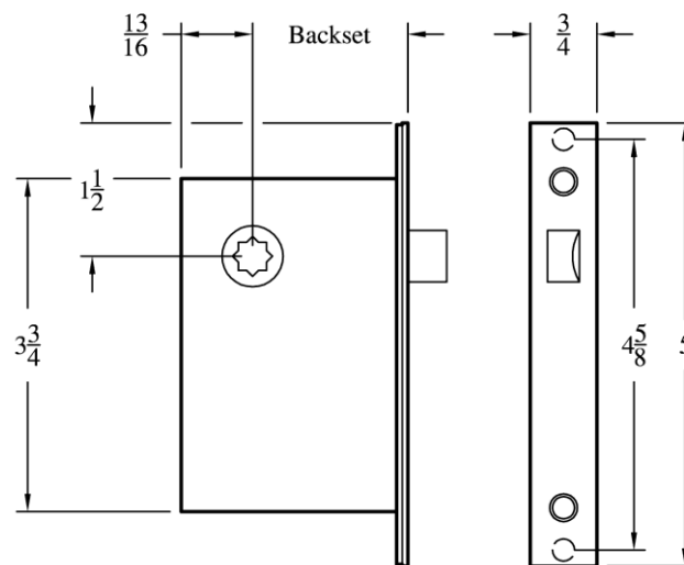
6525 Passage Latch Dimensions
