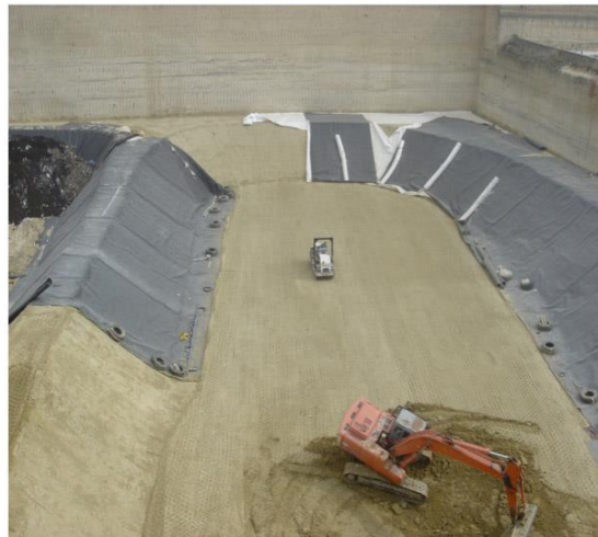
Fig. 4 Fasi di allestimento fondo della discarica – Lotto 3.
