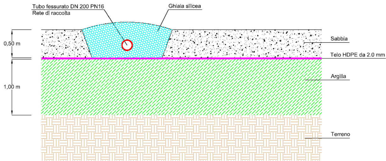
Fig.2 Sezione tipo del fondo della discarica con rete di captazione del percolato.
