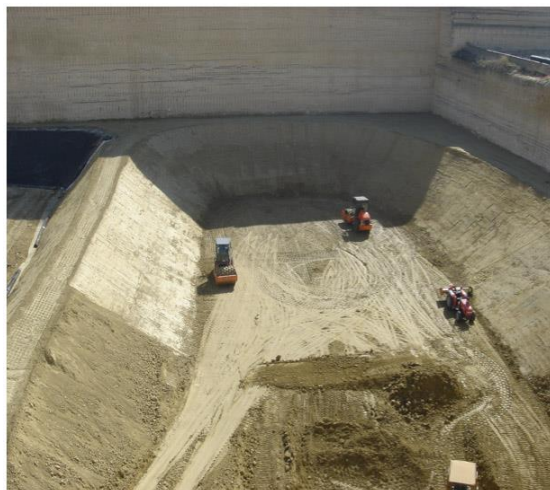
Fig. 3 Fasi di allestimento fondo della discarica – Lotto 3.
