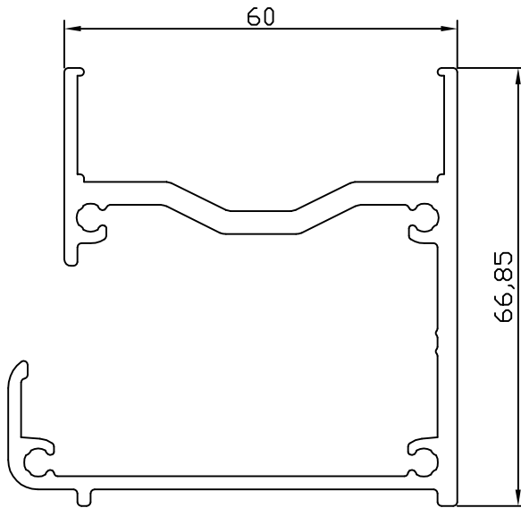
CANAL PARA REJILLA REF.54575
