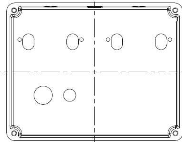
OD KIT 穴あけ加工図
