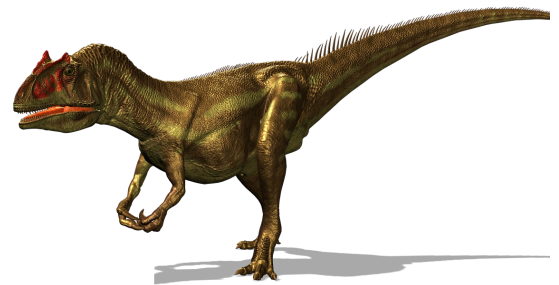
Allosaurus
