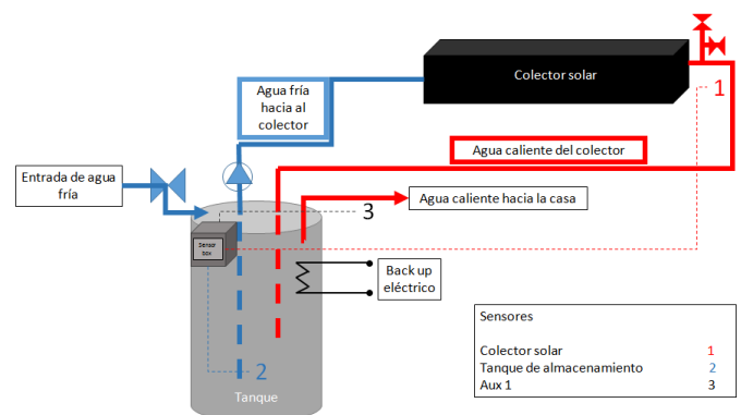
Figura IV-2 Sistema híbrido de calentamiento de agua solar
