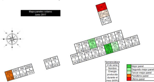
Figura IV-4 Desempeño por panel en Junio
