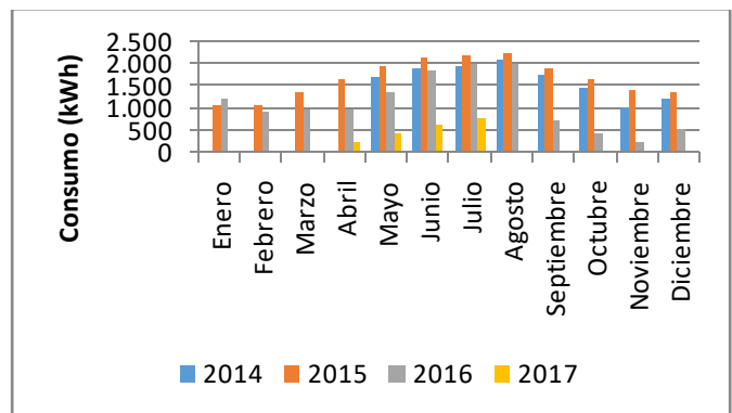
Figura V-1 Histórico de consume de energía eléctrica
