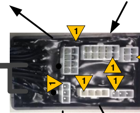
10 POS Molex 39-29-3106
