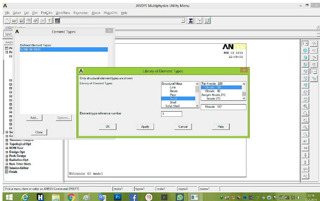
Şekil 1. Nitronic 60 model çeliğinin element türünün seçilmesi
