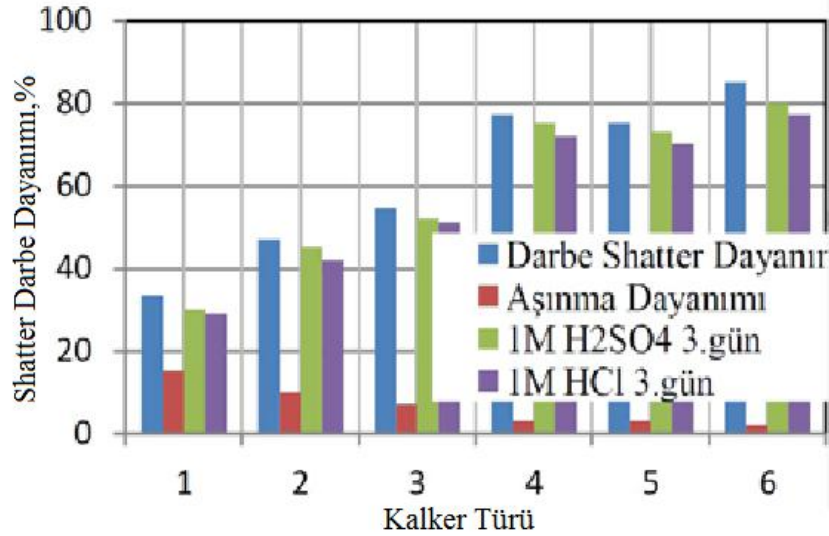
Şekil 3 % 4-7 gözenekli Şırnak kalkerini Kimyasal etkileşim sonrasındaki Darbe Dayanım ve Aşınma Direnci Kalker Türü:
