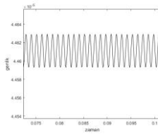
Şekil 5. Zaman tanım bölgesinde 75°C deki sönüm oranının titreşim karakteristiğine etkisi
