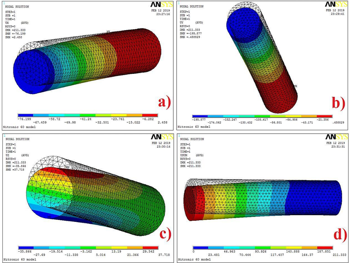
Şekil 10. Nitronic 60 model çeliğinin dik eksende a) x eksenindeki yer değiştirmesi b) y eksenindeki yer değiştirmesi c) z eksenindeki yer değiştirmesi d) yer değiştirme global vektör toplamları
