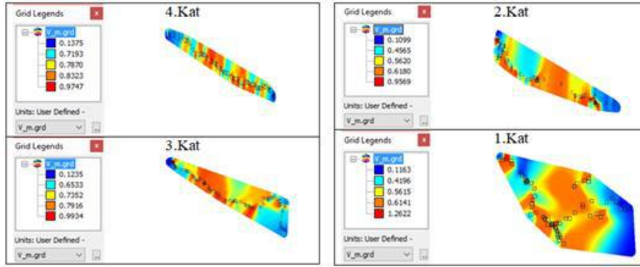
Şekil 17. Fen Edebiyat Fakültesi B Blok binasında 100 kHz - 8 GHz frekans aralığında ölçülmüş olan maksimum ve minimum elektrik alan şiddetinin değerleri ve 2 boyutlu haritalarıdır.
