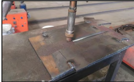
Şekil 1. Kaynak esnasında puntalanmış numune görüntüsü
