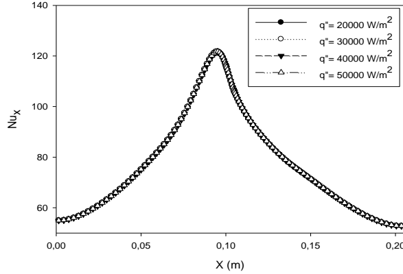
Şekil 4. Farklı ısı akılarının yerel Nusselt sayıları
