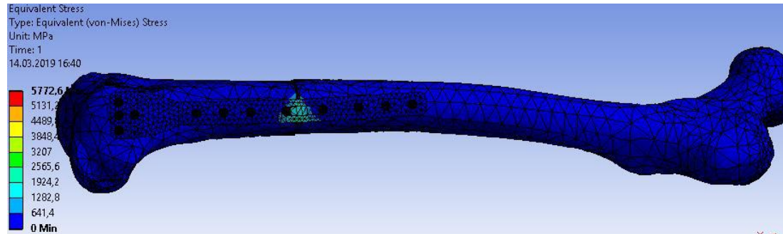
Şekil 4. Von-Mises gerilmeleri
