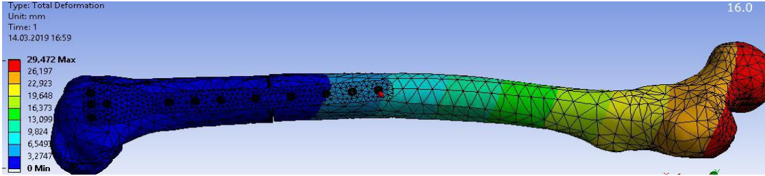
Şekil 7. Toplam deformasyon
