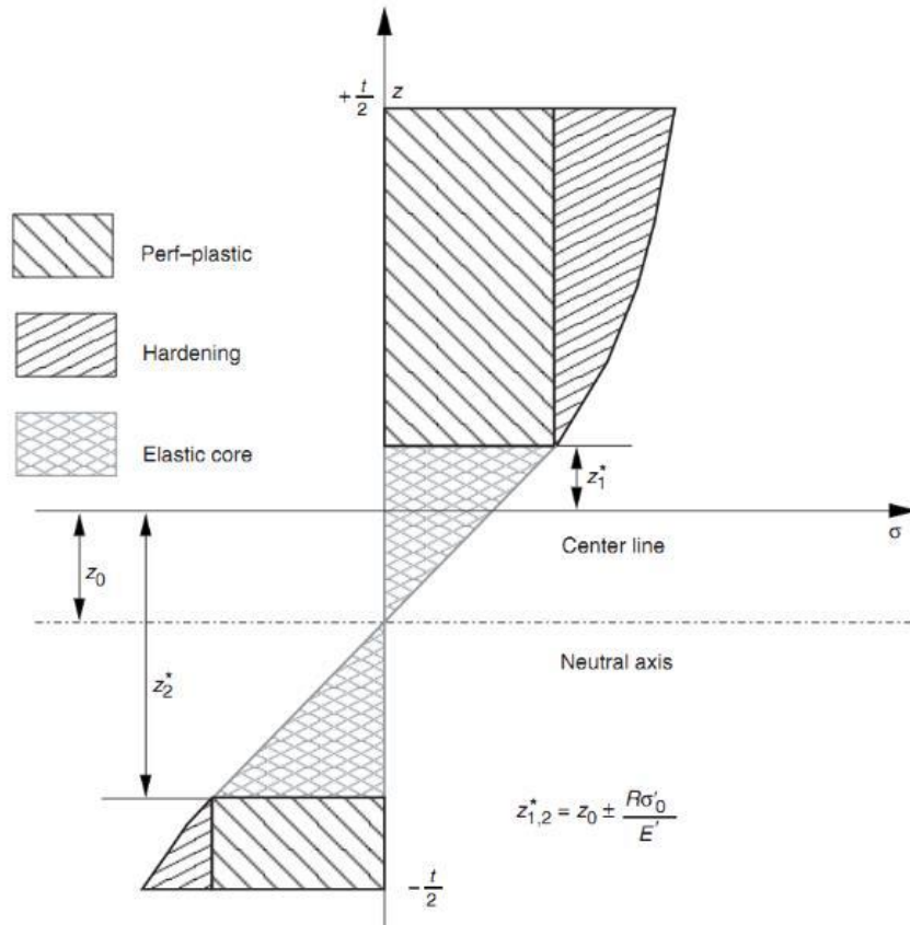
Şekil 6; Büküm Kesiti
