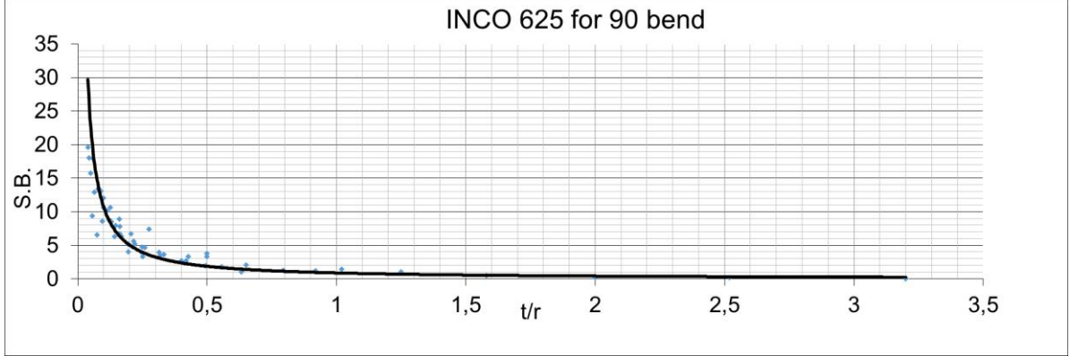
Şekil 5; Deneysel Sonuçlar
