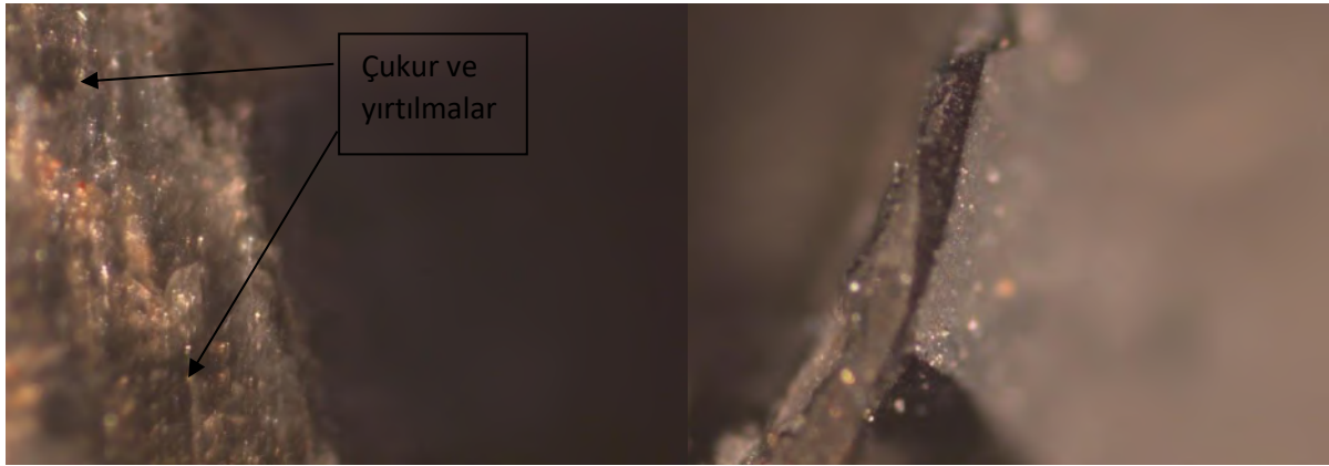
Şekil 65b. Takım aşınması Leika mikroskop görüntüleri.
