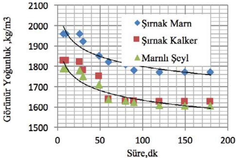
Şekil 2 Kimyasal etkileşim sonrasında Toz kalker dolgulu Epoksi Dolgu yoğunluk değişimi
