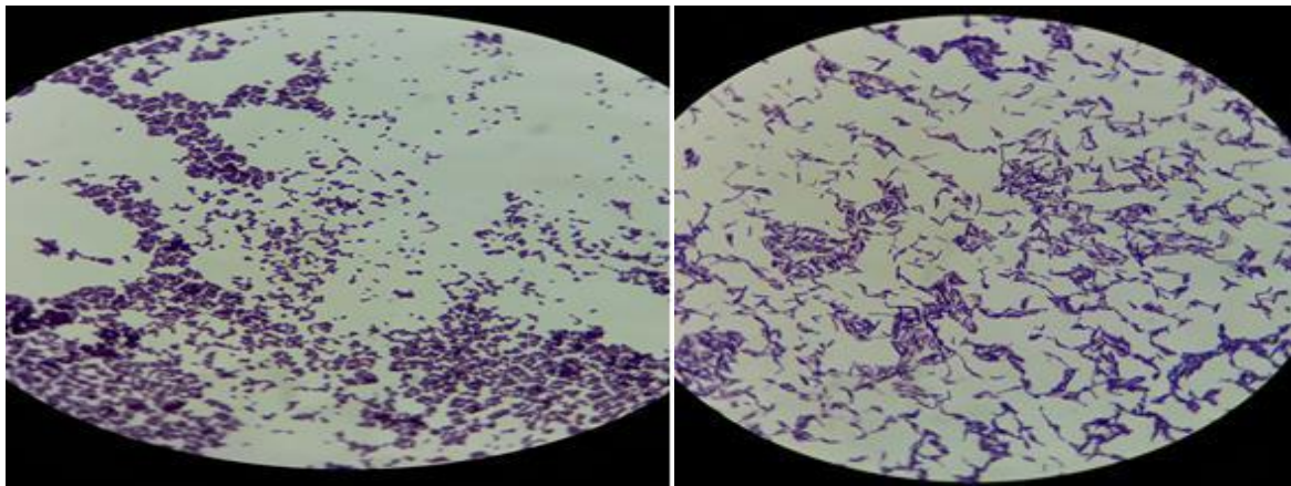
Şekil 2. LAB temsili mikroskop görüntüsü
