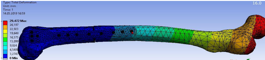
Şekil 7. Toplam defomasyon
