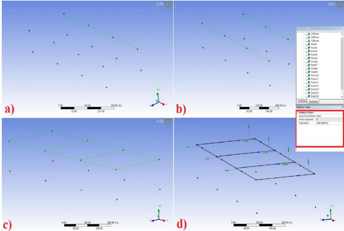
Şekil 5. İki katlı bina prototipinin a) 1.kat arka kirişin oluşturulması b) 1.kat ön kirişin oluşturulması c) 1.kat bütün kiriş tabakalarının birleştirilmesi d) Kiriş tabakalarının 6 eksende belirlenmesi ve gösterimi
