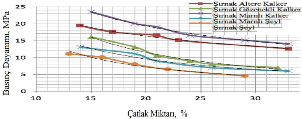
Şekil 3 % 14-37 çatlaklı Şırnak Kalker Türlerinin Kimyasal etkileşim sonrasındaki Basınç Dayanımı:
