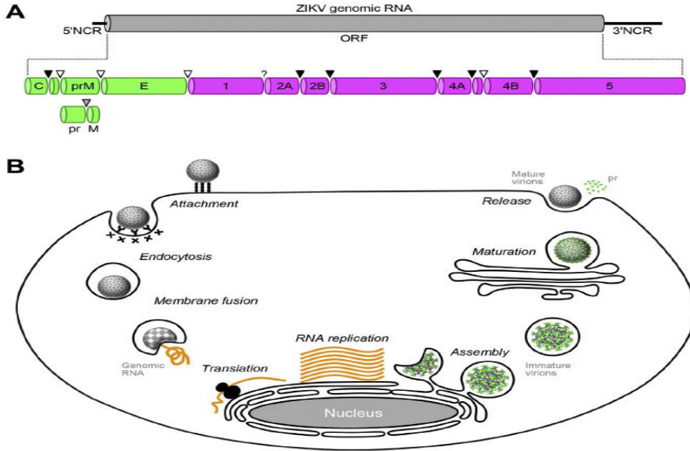
Şekil 1. ZIKV genom yapısı ve çoğaltma döngüsü. (A) ZIKV genomik RNA'sının şematik bir diyagramı. Viral genomda kodlanan tek açık okuma çerçevesi (ORF), ORF'nin altında tanımlanan üç yapısal (yeşil) ve yedi yapısal olmayan (mor) proteinler gösterilmiştir. (B) ZIKV'nin öngörülen yaşam döngüsü. Viral yaşam döngüsünün sekiz ana basamağı şunlardır: bağlanma, endositoz, membran füzyonu, çeviri, RNA replikasyonu, hücre toplanması, olgunlaşma ve salınma [5].
