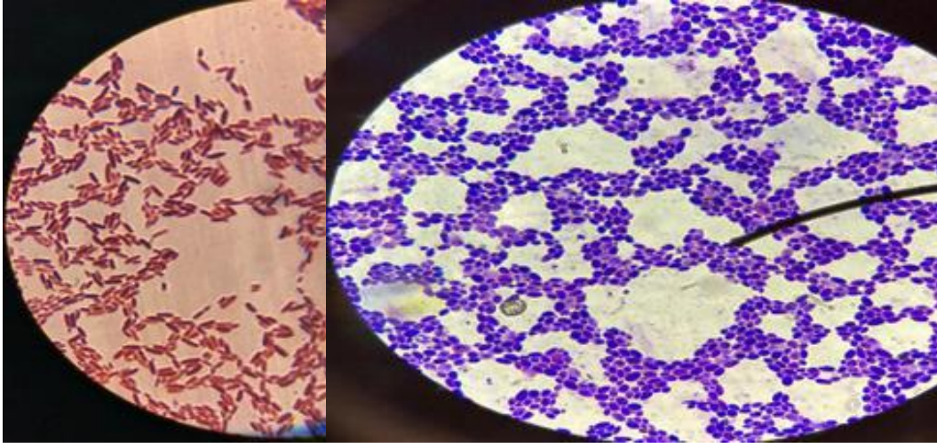
Şekil 4. Maya temsili mikroskop görüntüleri
