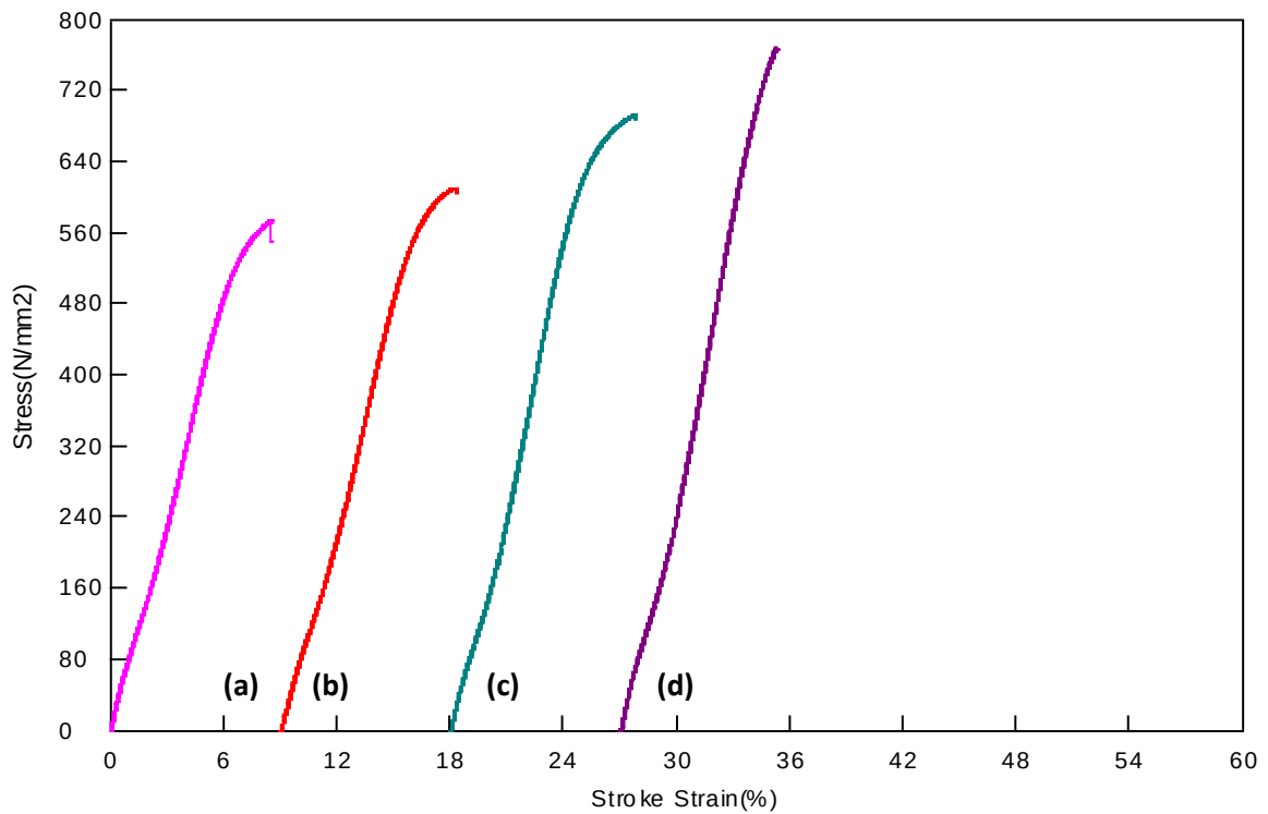
Şekil 2. 1400°C sinterleme sıcaklığında sinterlenen TM çelik numunelerin çekme eğrileri (a-Alařım 1, b-Alařım 2, c-Alařım 3 ve d-Alařım 4).
