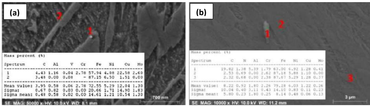
Şekil 3. 1400°C sinterleme sıcaklığında sinterlenen Alaşım 3 TM çelik numunenin SEM mikroyapı resimleri ( a-50000x b-10000 x)
