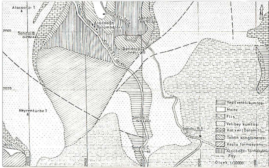
Şekil 4- Alacaagzı Yolunda ve Neyrentürbe Civarında Tipik Velibey Kumtaşı Serileri.
