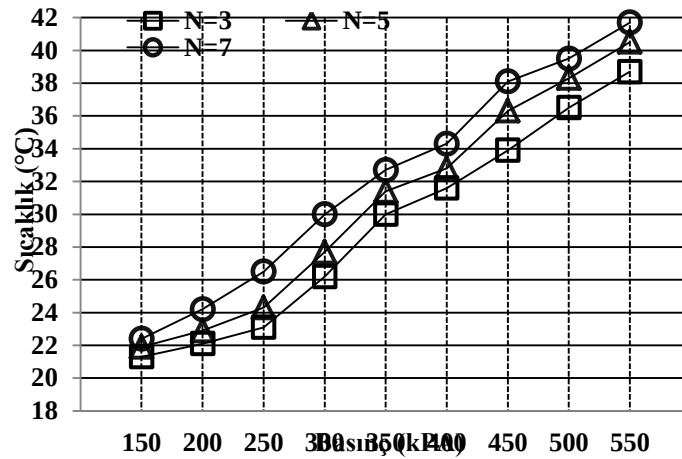
Şekil 5. Giriş Basıncı ile T_{sck} değişim grafiği
