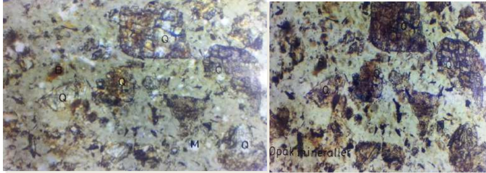
Şekil 13- Karbonifer Kumtaşına Ait İnce Kesitten Doğal Işıktaki (solda) ve Polarize Işıktaki Çekilmiş x176 Büyütmeli Mikrofotografılar.
