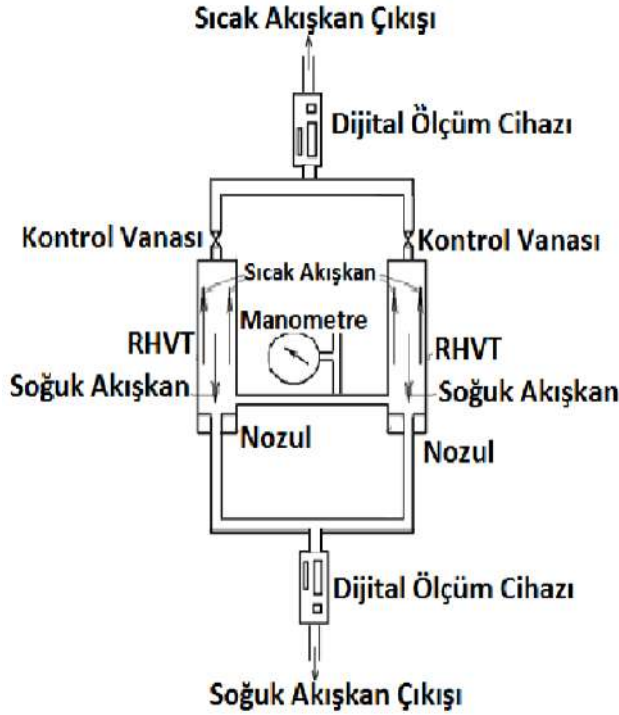
Şekil 2. Paralel Bağlı RHVT deneysel sistem
