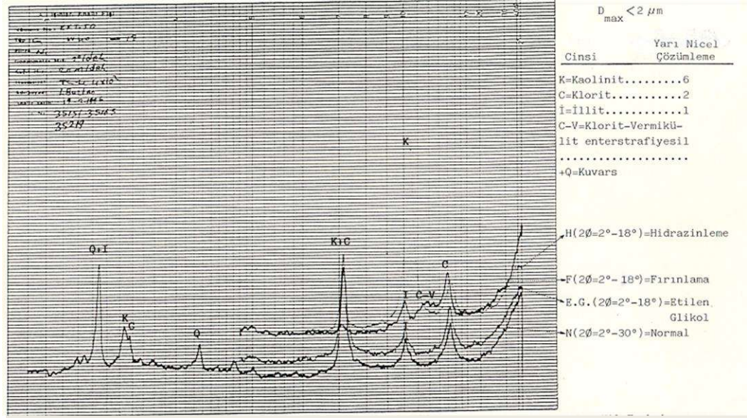
Şekil 17- Kandilli Açık İşletmesi Karbonifer Kumtaşının XRD Yöntemiyle Elde Edilen Kil Fraksiyonu Difraktogramı ( 2\theta = 2-30^\circ ) ve Çözümlemesi.
