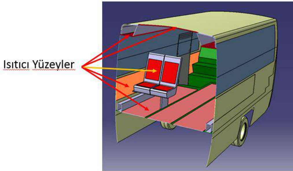
Şekil 2. Dokuma tekstil ısıtıcıların uygulandığı yüzeyler
