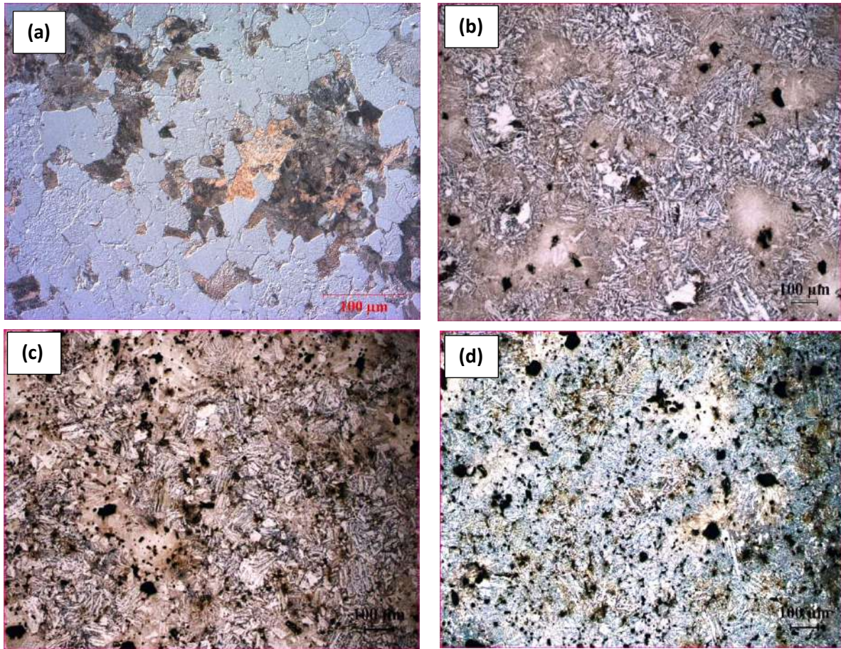
Şekil 1. 1400°C sinterleme sıcaklığında sinterlenen TM çelik numunelerin mikroyapı resimleri (100 x) (a-Alaşım 1, b-Alaşım 2, c-Alaşım 3 ve d-Alaşım 4).
