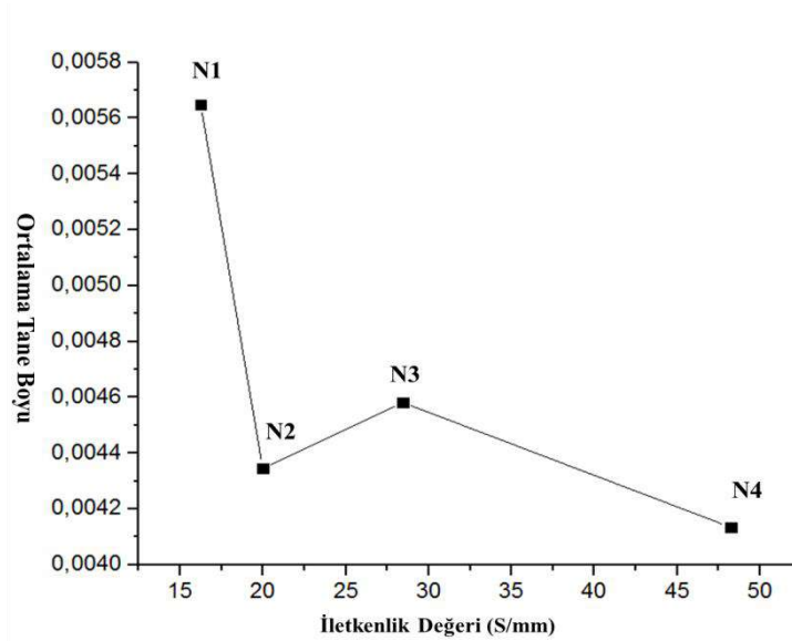
Şekil 7. Farklı ısıtıl işlem uygulanan numunelere ait iletkenlik değerleri ve tane boyutu
