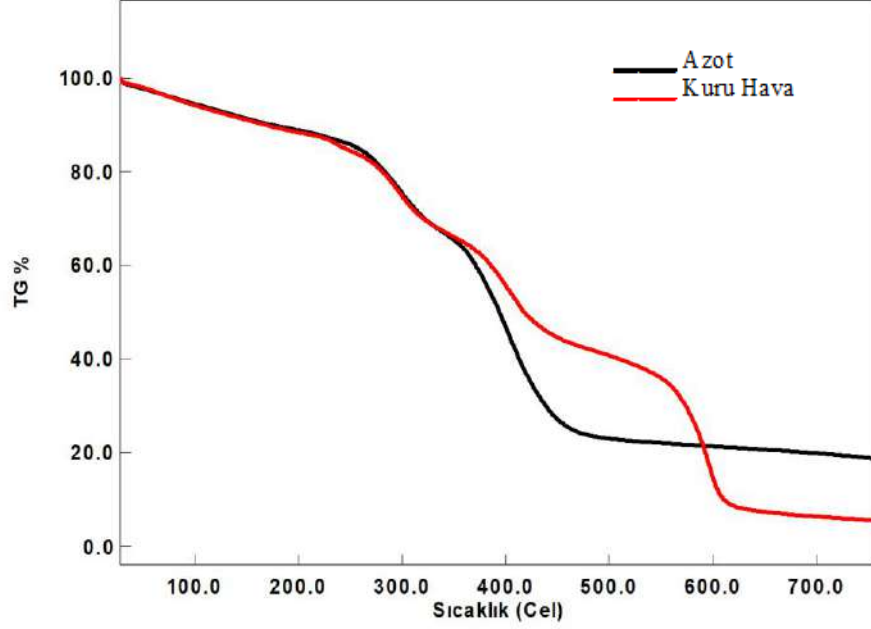
Şekil 4. A/MD-3:10/1 hidrojelinin farklı atmosferlerdeki (Kuru hava, Azot) %TG/Sıcaklık termogramı (20°C/dak ısıtma hızı)
