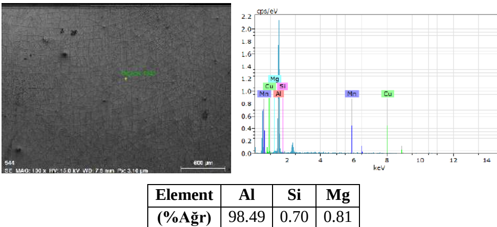
Şekil 5. N3 numunesi EDS analiz noktasının SEM fotoğrafı ve analiz sonucu
