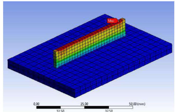
Şekil 2.2. Ansys analiz modeli ve sonuçlar.
