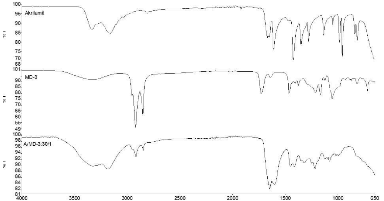
Şekil 3. Hidrojel sentezinde kullanılan monomerlerin (AAM ve MD-3) ve bir hidrojin karşılaştırmalı FT-IR spektrumları
