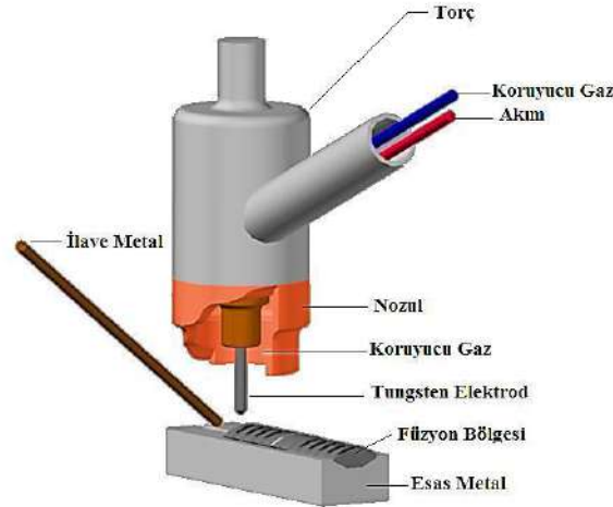
Şekil 2. GTAW yöntemiyle yapılan kaplama işleminin şematik görünümü.
