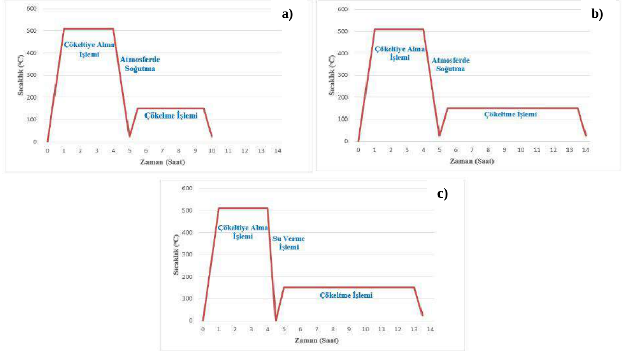
Şekil 1. 2024 Alüminyum alaşımına uygulanan ısıtma işlem ve yapay yaşlandırma işlemleri zaman-sıcaklık diyagramları a) N2 numunesi b) N3 numunesi c) N4 numunesi
