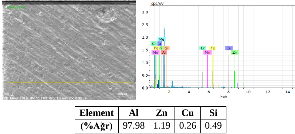
Şekil 3. N1 numunesi EDS analiz noktasının SEM fotoğrafı ve analiz sonucu
