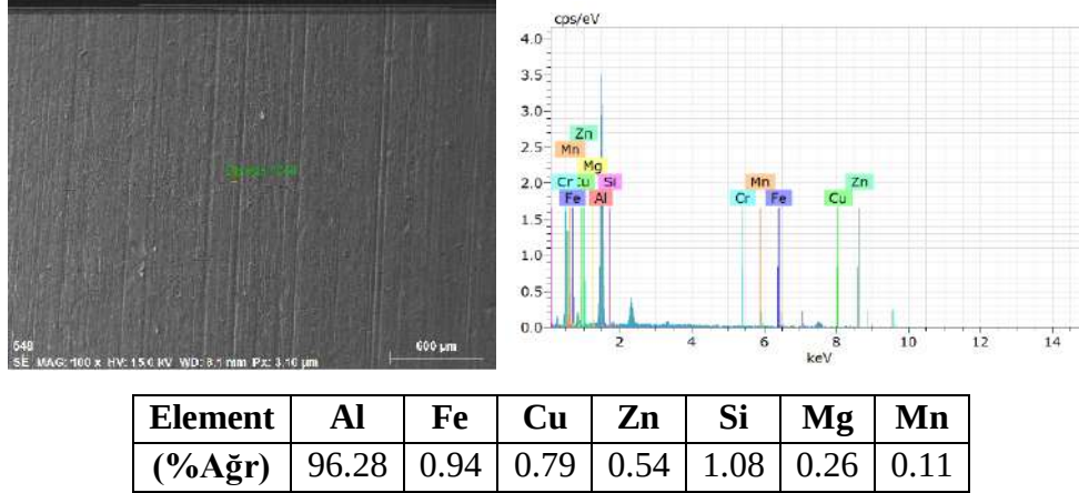
Şekil 4. N2 numunesi EDS analiz noktasının SEM fotoğrafı ve analiz sonucu
