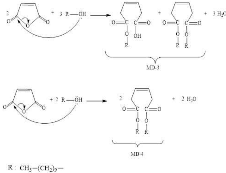
Şekil 1. Maleik anhidritin 1-dekanol ile modifikasyonu
