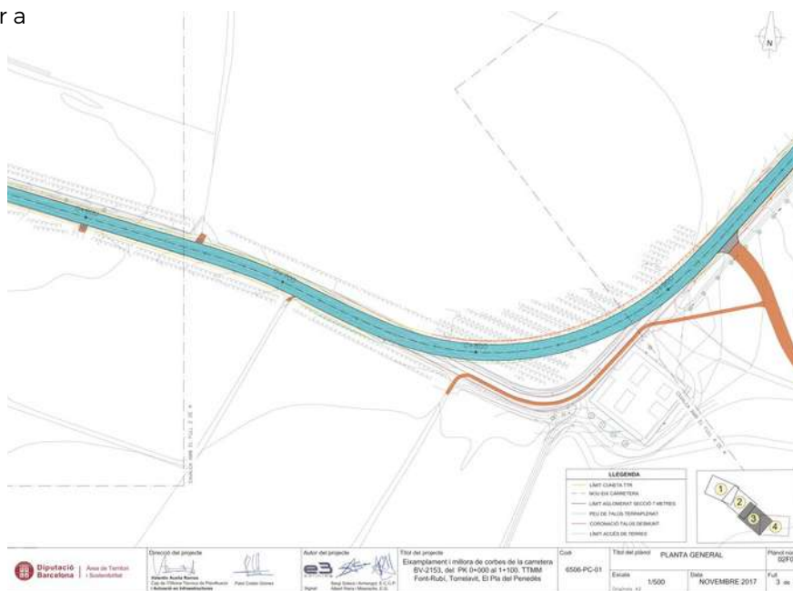
Croquis obra
