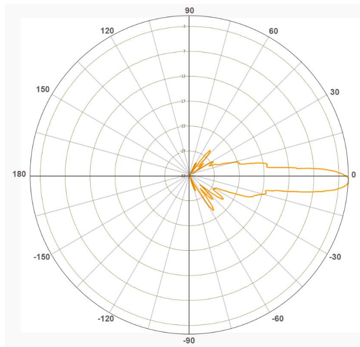
H-Plane Pattern (QAD 0529 - 65 SD)
