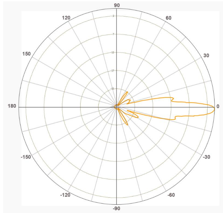
E-Plane Pattern (QAD 0529 - 65 SD)
