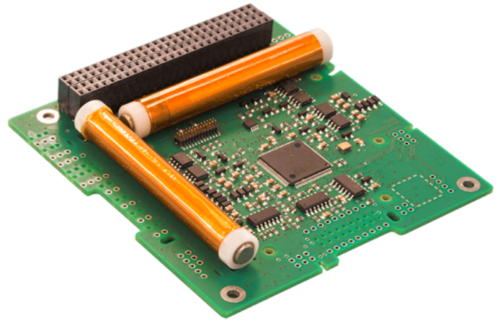
fig(2) Magnetorquer
