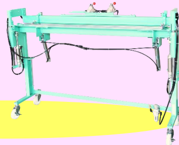
縁無畳製作支援機:ツイスト 縁無表曲機:スリムバンダー
