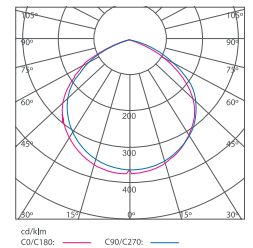
K10143 150W
