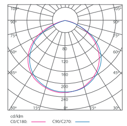
K10140 30W
