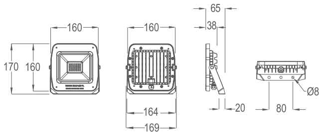
K10141 50W
