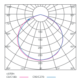
K10141 50W
