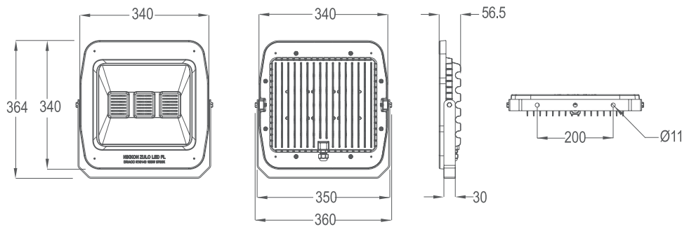
K10143 150W
