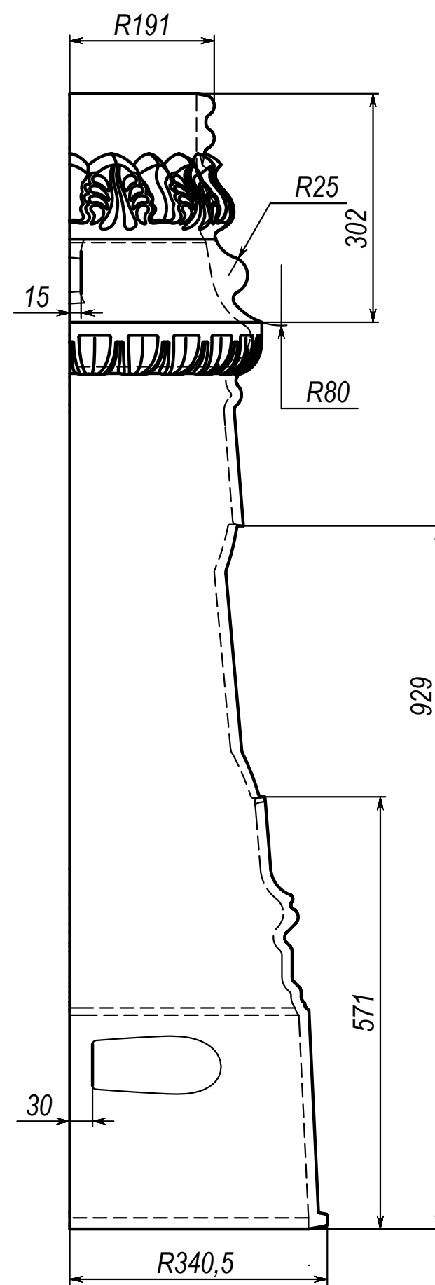
Цоколь Ц7 Масса 125,6 кг
