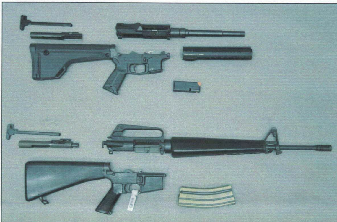
Abbildung 5: Vergleichsansicht rechte Seite, oben die halbautomatische „The 9ers-Sport-C“, unten die vollautomatische „AR15“, beide zerlegt in die jeweiligen Hauptgruppen
